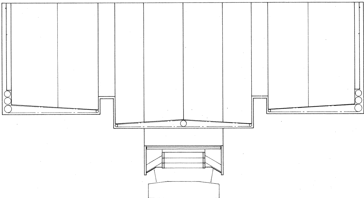
PROSPEKTZEICHNUNG STIFTSKIRCHE, BAD GANDERSHEIM M = 1 : 25
